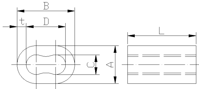
寸法表
